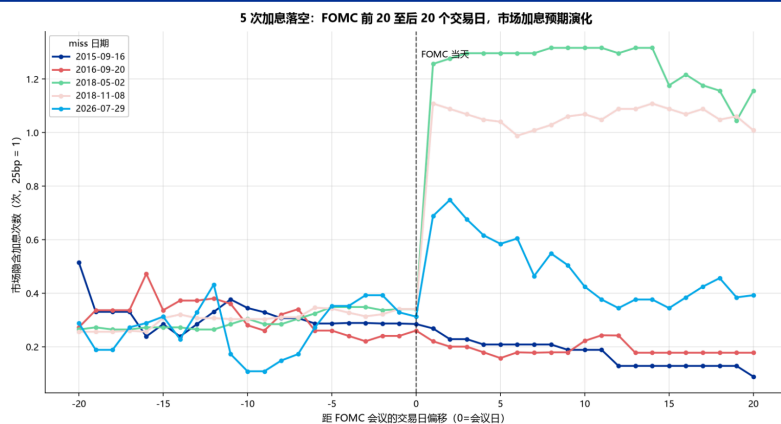
图表 12：加息落空后，FOMC 会议前后市场对下次会议加息预期的演变
